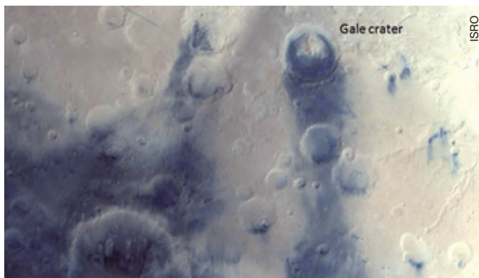
▲ Снимок 155-километрового кратера Гейл (Gale). Возраст этой ударной структуры оценивается в 3,5-3,8 млрд лет.
