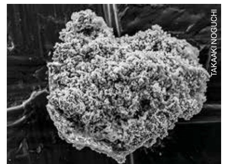
▼ Электронная микрофотография одиночной частицы кометной пыли, найденной в антарктическом льду.
