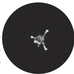
◀ Зонд Philae после отделения, запечатленный камерой OSIRIS аппарата Rosetta 12 ноября 2014 г. в 10:23 GMT (указано бортовое время).
