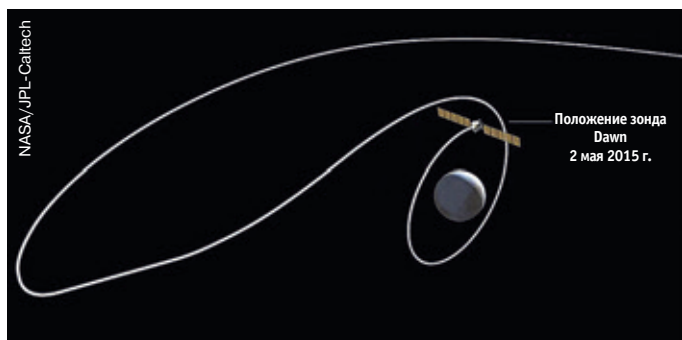
▲ Космический аппарат Dawn должен произвести серию сложных маневров с помощью бортовых ионных двигателей, чтобы к маю достичь первой рабочей орбиты вокруг Цереры, после чего двигательная установка будет выключена до начала следующей фазы научных исследований. (Размер Цереры на этом рисунке преувеличен по сравнению с размерами орбиты.)
