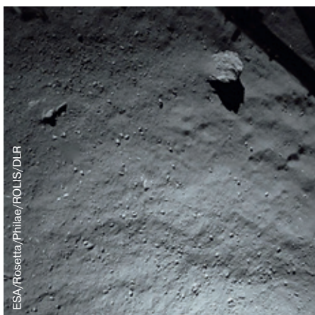
▲ Снимок поверхности ядра с высоты 40 м, переданный камерой ROLIS посадочного модуля. Валу в правой верхней части снимка имеет поперечник около 5 м.
