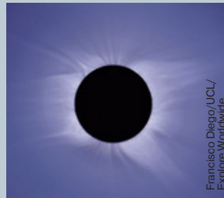
▲ Полное солнечное затмение 20 марта 2015 г. крупным планом
