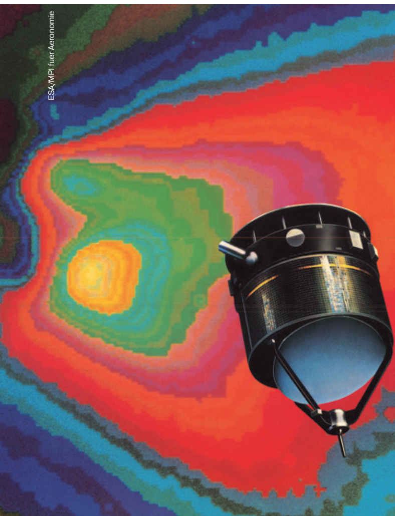
▲ Снимок ядра кометы Галлея, полученный космическим аппаратом Giotto и сильно разочаровавший Маргарет Тэтчер.
