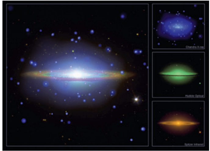
▲ Галактика M104 «Сомbrero» — один из крупнейших и ближайших к нам членов скопления Девы (от нее нас отделяет 28 млн световых лет). Это ее изображение составлено по данным съемки в рентгеновском диапазоне (обсерватория Chandra, показаны голубым цветом), видимом свете (Hubble, зеленый цвет) и в инфракрасных лучах (Spitzer, оранжевый цвет). Каждый спектральный диапазон отображает определенные особенности галактической структуры.
