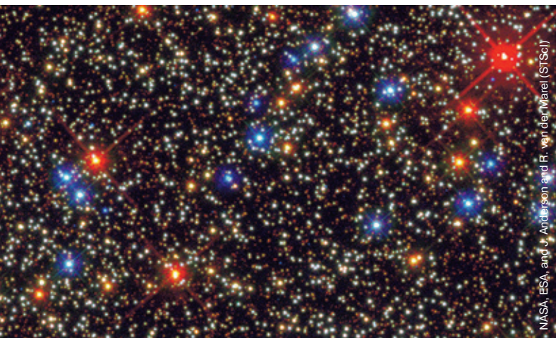
▲ Шаровое звездное скопление \omega Центавра открыл древнегреческий астроном Птолемей почти 2 тыс. лет назад, однако он посчитал его простой звездой, поэтому в более поздних каталогах оно получило «звездное» обозначение. На самом деле оно содержит около 10 млн звезд.
