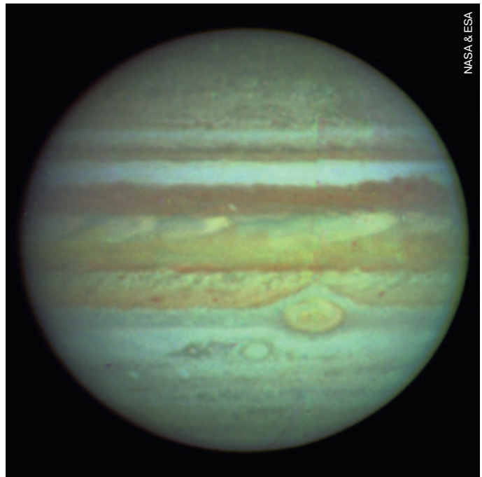
▲ «Зеленый» Юпитер на снимке Камеры широкого поля телескопа Hubble. На фотографиях, предназначенных для публикации, цвет планеты был откорректирован.
