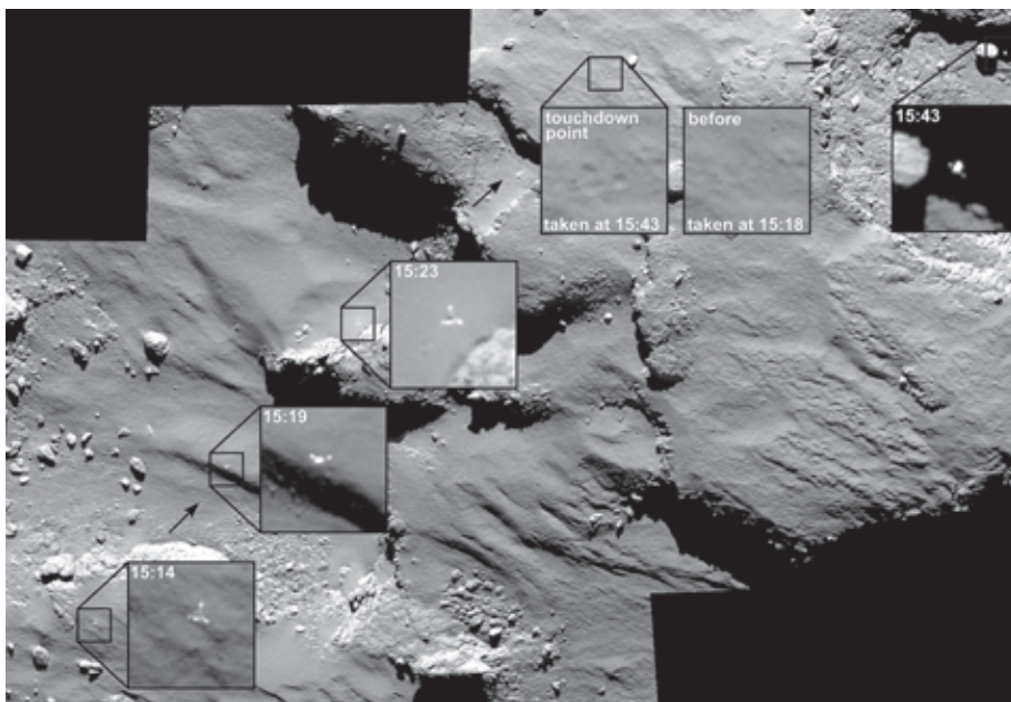
▲ Полет Philae над ядром. Модуль совершил, по меньшей мере, два «прыжка». Его окончательное местонахождение определено с точностью до 100 м.
