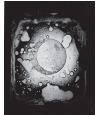
▲ Один из первых снимков Луны, полученный Джоном Дрейпером 26 марта 1840 г. на собственной обсерватории в Нью-Йорке (самый первый снимок, судя по всему, не сохранился). Поскольку фотопластинка устанавливалась в главном фокусе рефлектора, изображение получилось зеркально отраженным.
