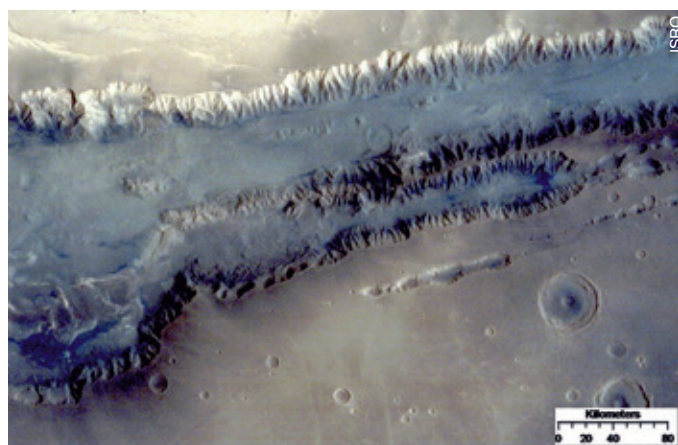
▲ Новые фотографии, представленные ISRO, демонстрируют возможности камеры MCC космического аппарата «Мангальян», способной с различных расстояний получать снимки общего плана и детальные изображения марсианской поверхности. Большой Каньон, или Долина Маринера, представляет собой самую большую из подобных структур в Солнечной системе — его длина превышает 4 тыс. км, а глубина достигает 7 км. Его общий вид сфотографирован 5 декабря 2014 г. с высоты 24 тыс. км, а отдельные снимки его участков были сделаны 28 января с высоты 5800 км.
