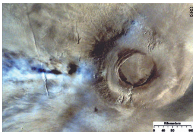
▲ Вулкан Арсия с окружающими его грядками облаков, сфотографированный 4 января с высоты 10 700 км. Он имеет высоту около 16 км и диаметр у основания 435 км.
