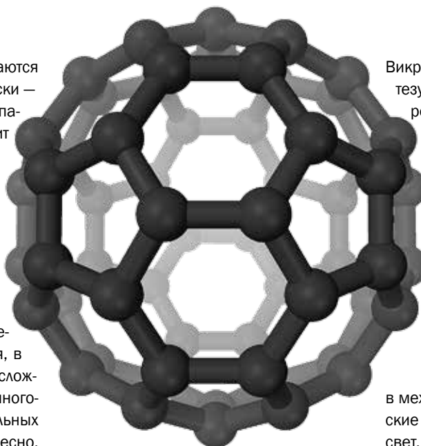
▲ Молекула фуллерена C 60 состоит из двенадцати правильных пятиугольников, окруженных шестиугольниками общим числом 20.
