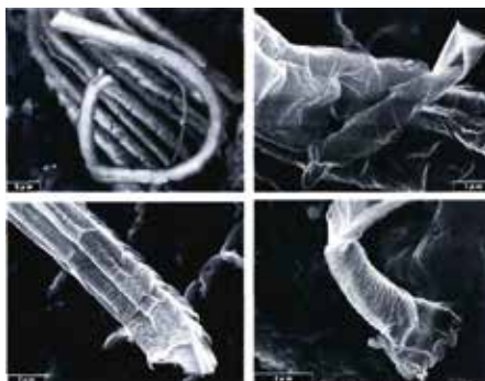
▲ Псевдоморфозы в метеорите Оргей по А.Ю.Розанову
